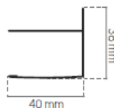
2-teilige-Schiebetür, Schiebeelemente aushängbar
