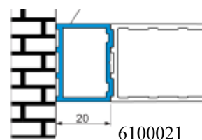
Erweiterungsprofil.
