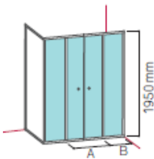
4-teilige-Schiebetür, Schiebeelemente aushängbar
