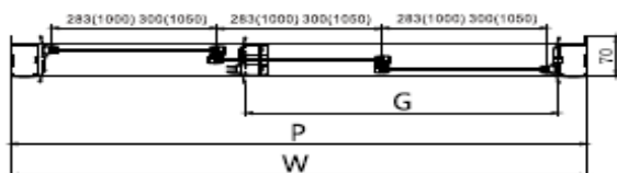
3-teilige Schiebetür, 4 mm ESG Sicherheitsglas
