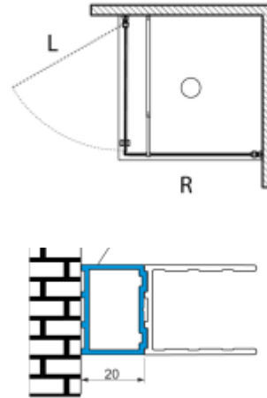
Erweiterungsprofil (Artikel Nr. 6100021)
