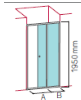
2-teilige-Schiebetür, Schiebeelemente aushängbar
