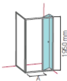
Faltdür, vorgerahmt, 4mm ESG Sicherheitsglas
