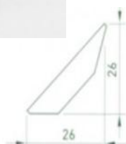
21301 Dreikantleiste P-26
